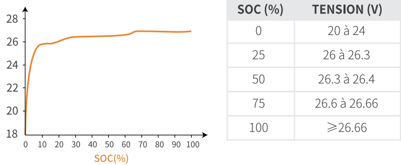
TENSION (V)
